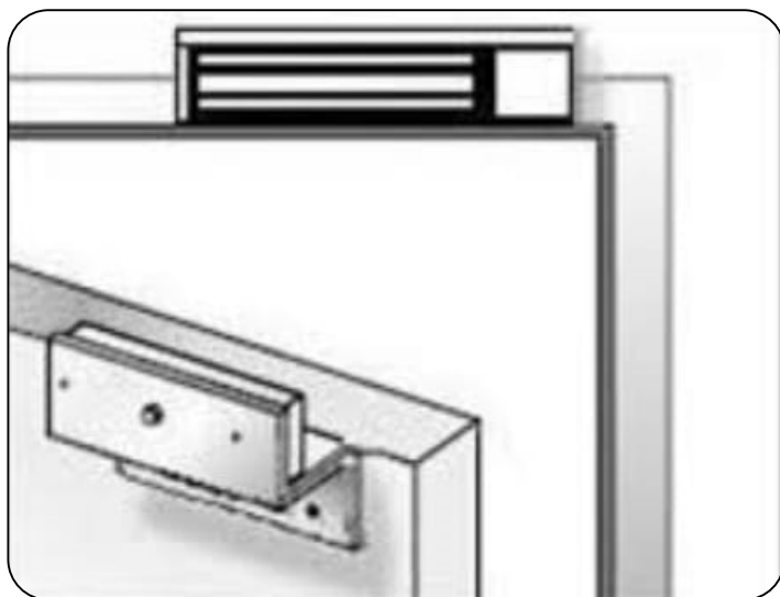
LZ-bracket for inswing door
